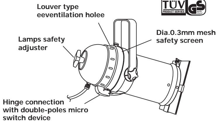
PAR 64 with TUV approval (EN60598-2-17)
